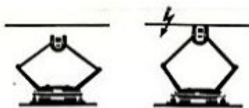
Kohlewechsel Replacing carbon brushes Changement des balais
